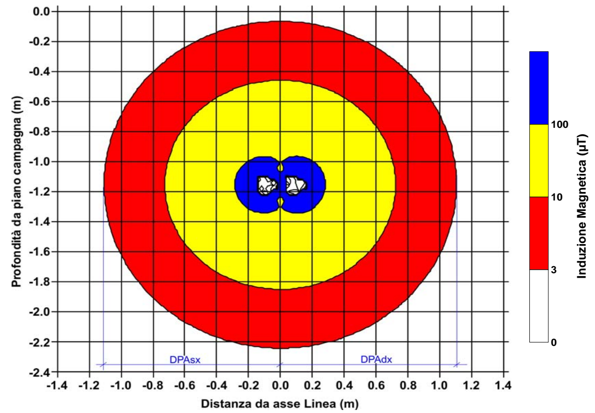
Induzione magnetica su un piano verticale perpendicolare alla linea nell'ipotesi di carico pari a 295 A per ciascuna terna. DPAdx = 1.10 m; DPAsx = -1.10 m
