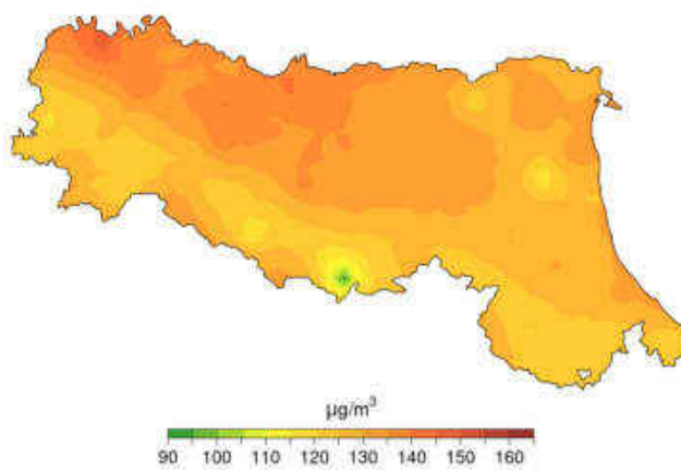
Figura 98. Concentrazione media annuale di O 3 (µg/m 3 ) nello scenario base (2017)
