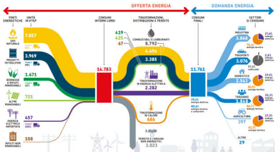
Figura 49> Rappresentazione diagrammatica del BER dell'Emilia-Romagna nel 2020 (diagramma di Sankey)
