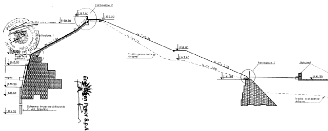
Figura 3 – sezione tipo a destra dello sfioratore
