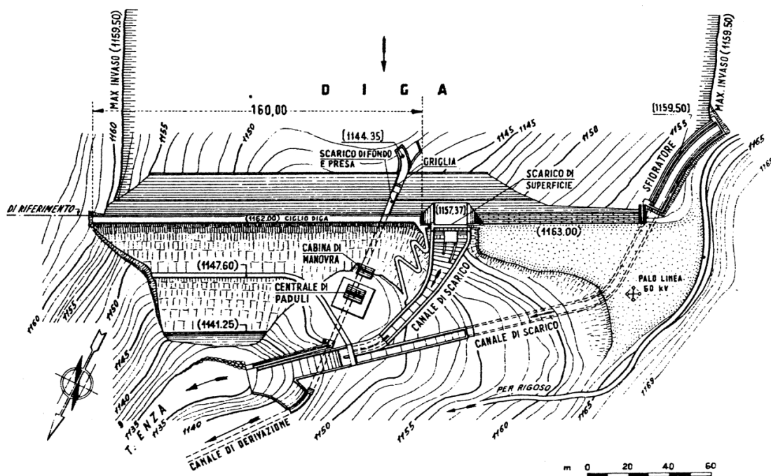
Figura 2 - Planimetria della diga e degli organi di scarico
