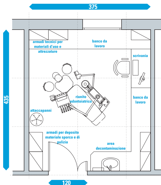
Fig. 4f AMBULATORIO ODONTOIATRICO (schema interpretativo della Norma di accreditamento regionale) 16mq
