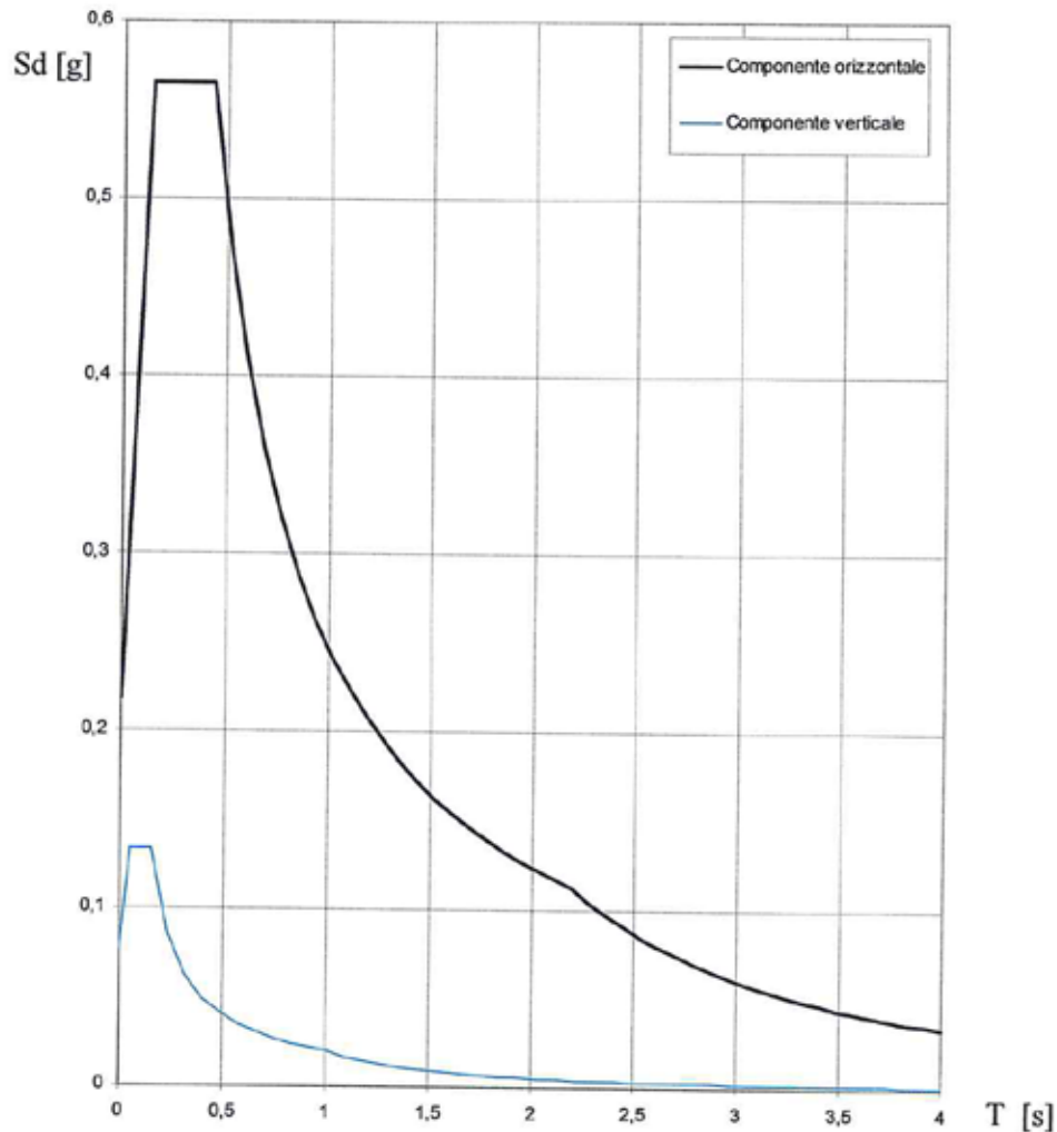
Spettri di risposta (componenti orizzontale e verticale per lo stato limite: SLV (da NTC 2008 vers. 1.03)
