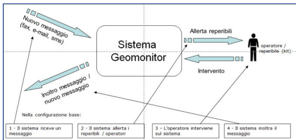
Figura 3-9 Schema di funzionamento.
