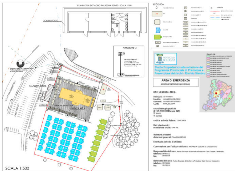
Figura 4-4 Schema rappresentativo dell'allestimento di un possibile campo di accoglienza.
