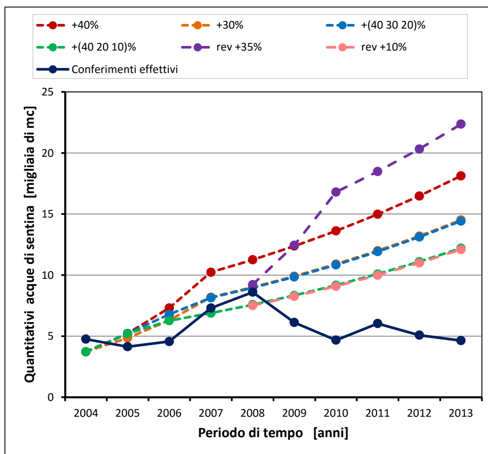
Figura 6.4 - Confronto scenari di produzione/quantitativi conferiti delle acque di sentina
