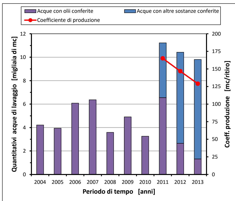
Figura 5.4 - Andamento annuale delle acque di lavaggio gestite
