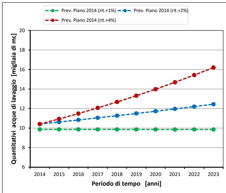
Figura 6.6 - Scenari di produzione delle acque di lavaggio
