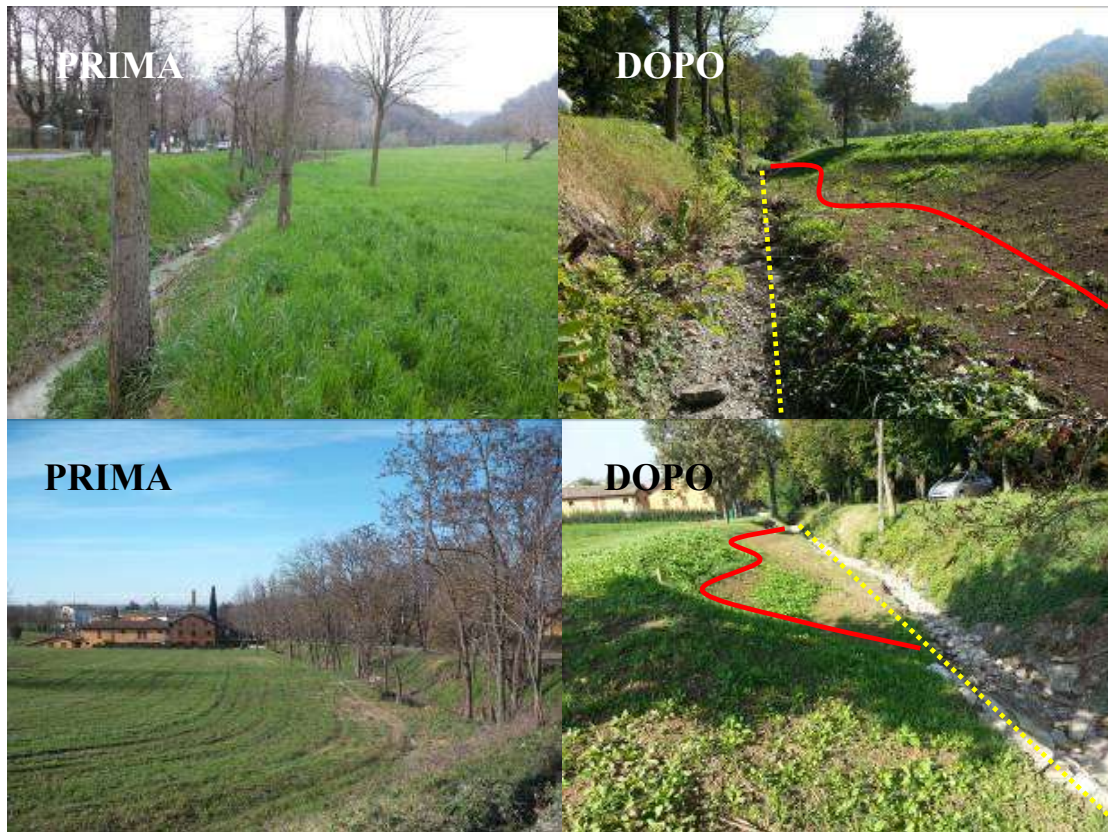
Figura 11 - Esempio di creazione di piana inondabile in un corso d'acqua non arginato mediante abbassamento del piano campagna (rio Bianello, Comune di Quattro Castella in Provincia di Reggio Emilia). Anche questo intervento, mostrato nelle immagini subito dopo la realizzazione dei lavori, fa parte delle azioni sviluppate nell'ambito del Progetto Europeo LIFE+ RII, come quello descritto in Figura 10. (linea gialla: sponda originale; linea rossa: sponda arretrata mediante sbancamento dell'area perifluviale). Intervento realizzato dal Consorzio di Bonifica dell'Emilia Centrale (RE). Foto: Marco Monaci.
