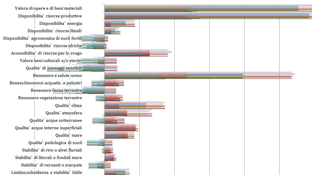
Figura. Stima della variabilità degli indici di impatto sui ricettori ambientali al variare dell'assegnazione finanziaria ai singoli obiettivi specifici. Per ciascun ricettore si hanno 46 linee, corrispondenti ai vari scenari alternativi considerati. Nonostante la valutazione sia ancora qualitativa, l'impatto sul ricettore può essere pensato come un impatto migliorativo (beneficio) se la linea è nel semiasse positivo, nella parte destra del grafico, mentre come un impatto negativo (danno) se la linea si trova nel semiasse negativo, nella parte sinistra del grafico.
