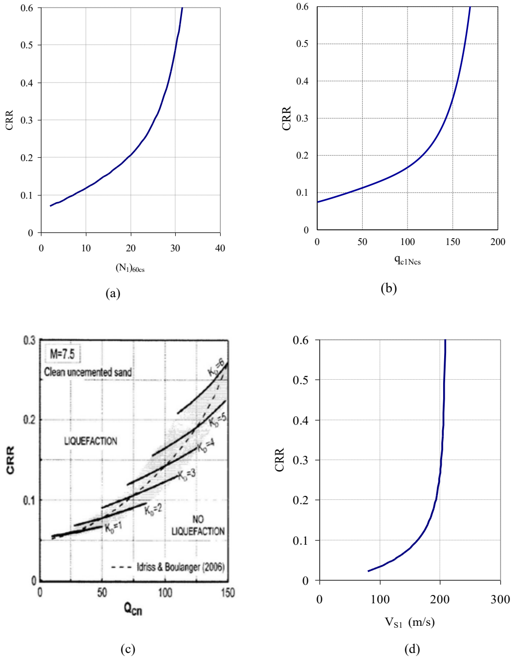
Figura 2 – Carte per la stima della resistenza normalizzata alla liquefazione CRR di un terreno sabbioso saturo sulla base dai risultati di prove SPT (a), CPTe (b), DMT (c) (Marchetti, 2015) e da profili di V_s (d)
