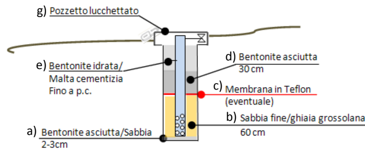
Figura 7: Schema riempimento intercapedine foro-sonda
