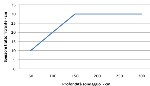
Figura 6: Diagramma profondità/tratto filtrante
