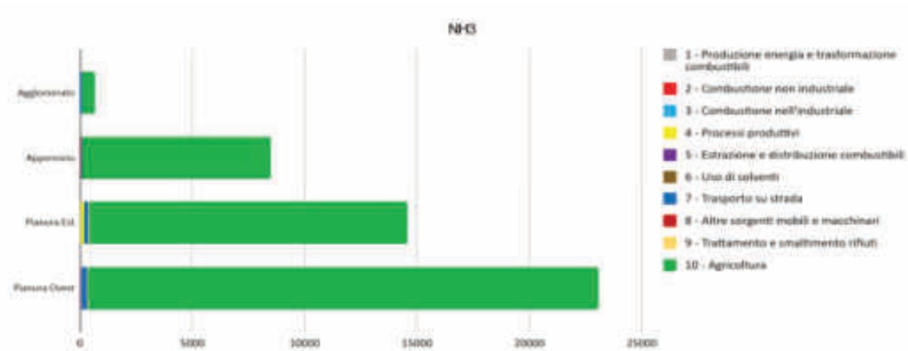
Fig. 28: Ripartizione per macrosettor dei contributi emissivi di NH3 per zone e agglomerato
