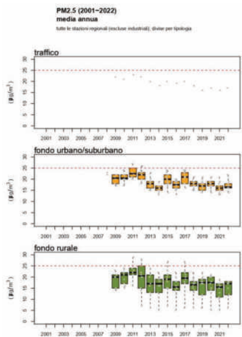
Fig. 10: Andamento della concentrazione media annuale di PM2.5 dal 2008 al 2022. La linea rossa indica il valore limite annuale ( 25 \mu\text{g}/\text{m}^3 ). I valori rilevati ogni anno dalle stazioni da traffico (in alto), di fondo urbano e suburbano (al centro) e di fondo rurale (in basso) sono rappresentati come box plot. Ciascun box rappresenta l'intervallo tra il 25° e il 75° percentile dei valori medi annuali ed è evidenziata la linea della mediana. Le linee verticali rappresentano il massimo e minimo. I punti contenuti in ciascun box forniscono una indicazione del numero e del valore dei dati che formano la distribuzione rappresentata dal box
