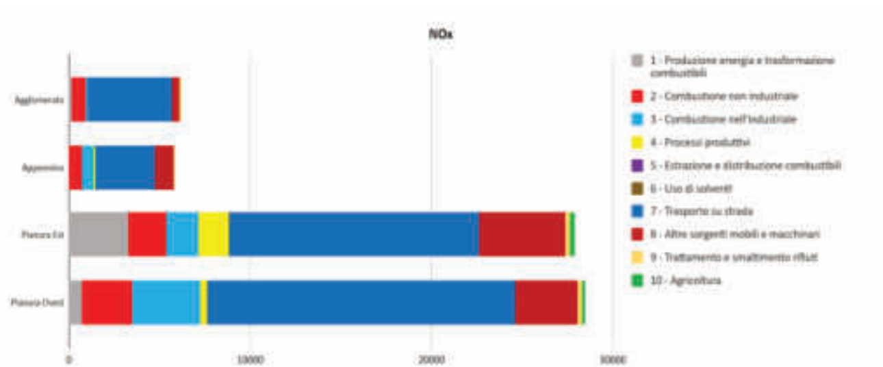
Fig. 27: Ripartizione per macrosettor dei contributi emissivi di NOx per zone e agglomerato
