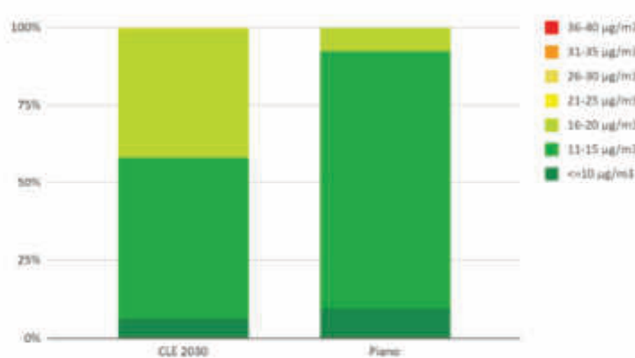
Fig. 113: Percentuale di popolazione esposta a diverse concentrazioni di NO 2 negli scenari CLE2030 e piano
